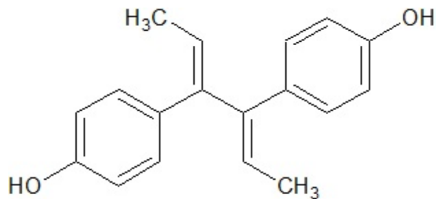
( trans-trans )-form
